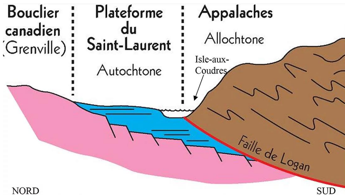
Figure 3. Coupe géologique à la hauteur de Charlevoix montrant la relation entre les Appalaches et le Bouclier canadien. L'île aux Coudres serait située juste à droite de la faille de Logan dans le fleuve.
